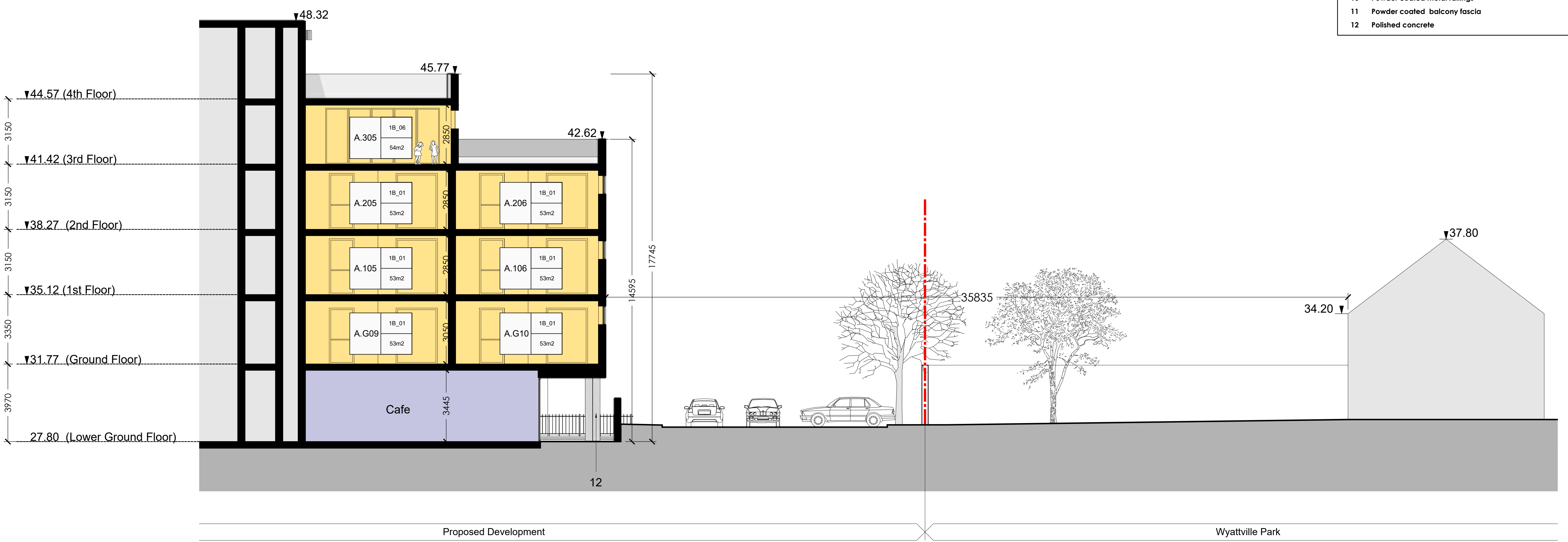
Section A-A (Building A) Scale 1:100@A0
